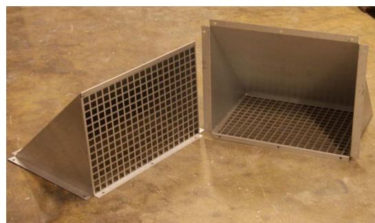
Bild 5: Intags-/avluftshuv 500x400
